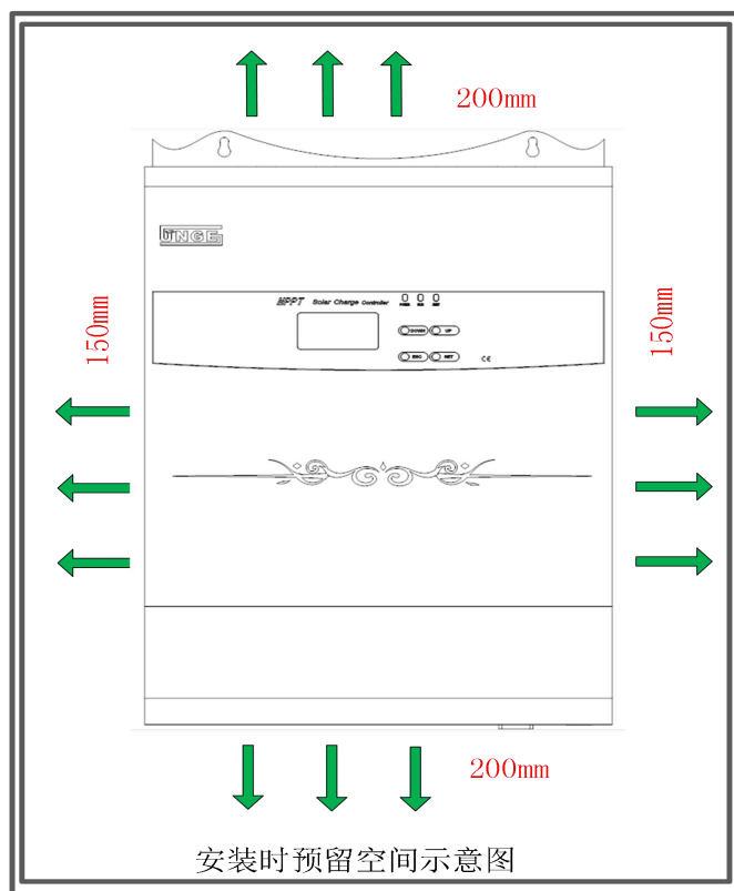
图 3-1 设备安装四周预留空间图
