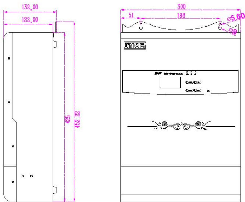
图 8-1 JN-HV 50A 控制器安装尺寸图(mm)
