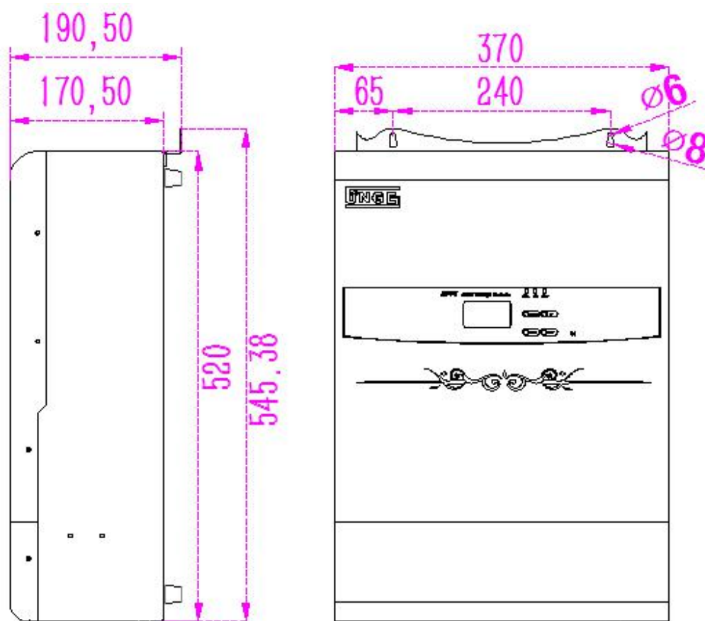
图 8-2 JN-HV 100A 控制器安装尺寸图(mm)
